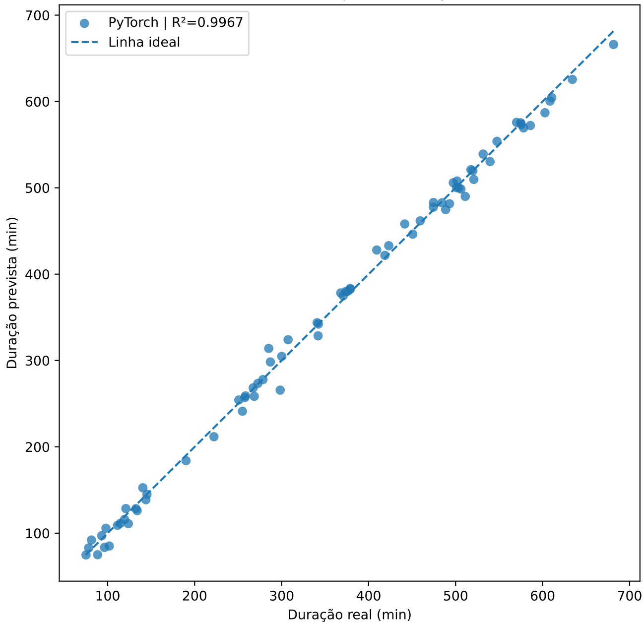
Valores reais vs. previstos - PyTorch
